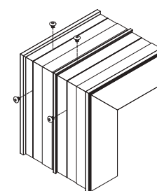
Tham khảo ghép góc cánh 45° ke vĩnh cửu (Vít lục giác)
