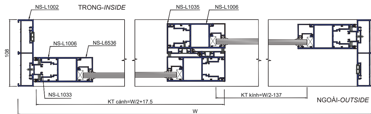
CHI TIẾT 2-2
