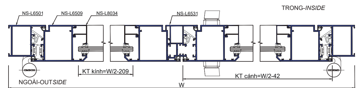
CHI TIẾT 3-3
