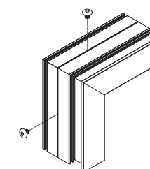
Tham khảo ghép góc cánh 45^\circ ke vĩnh cửu (Vít lục giác)
