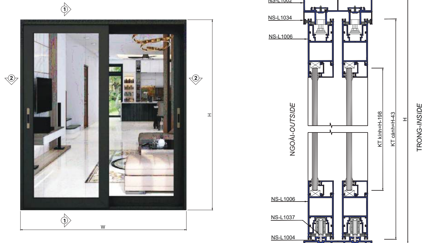
Cửa đi lùa 2 cánh (ray bằng)
