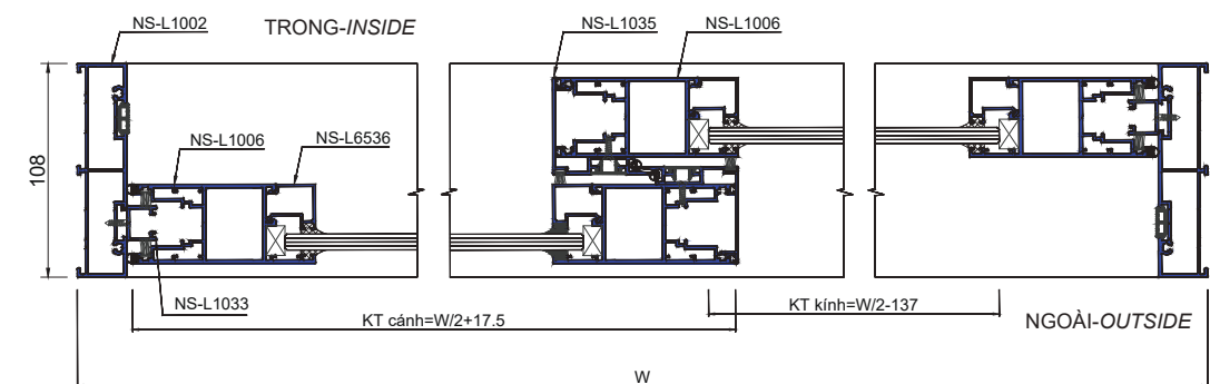
CHI TIẾT 3-3
