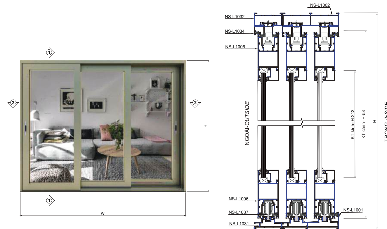
CHI TIẾT 1-1
