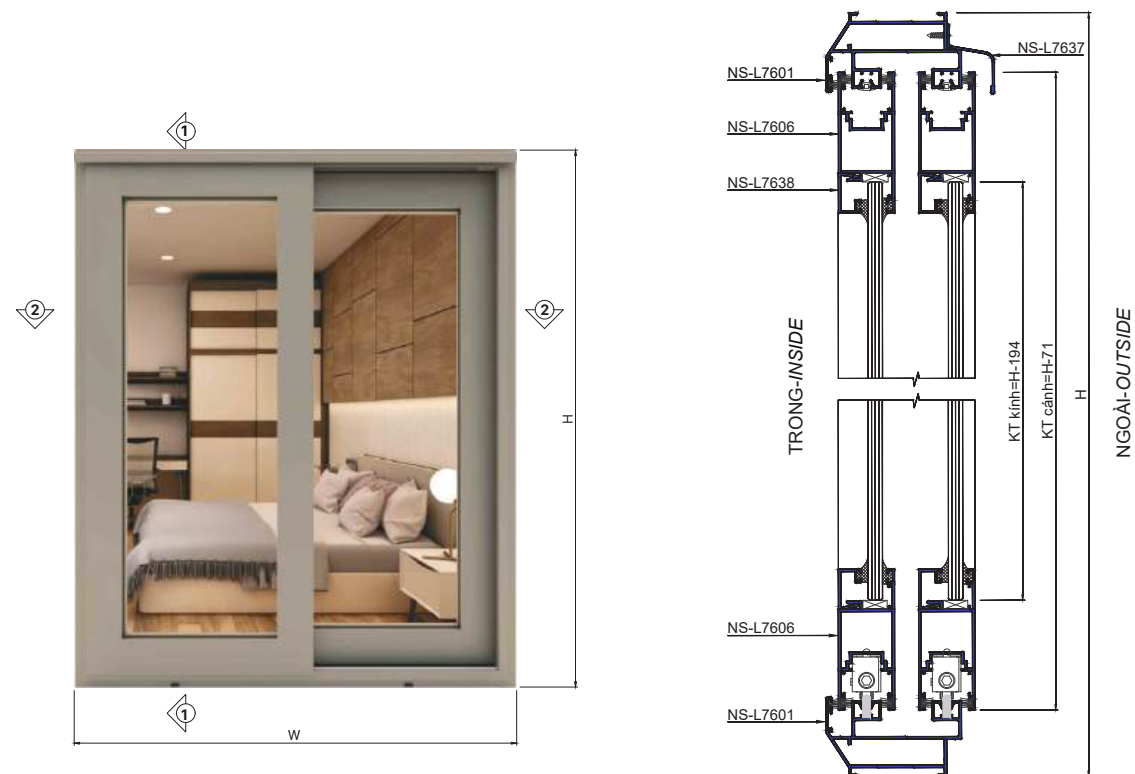
CHI TIẾT 1-1
