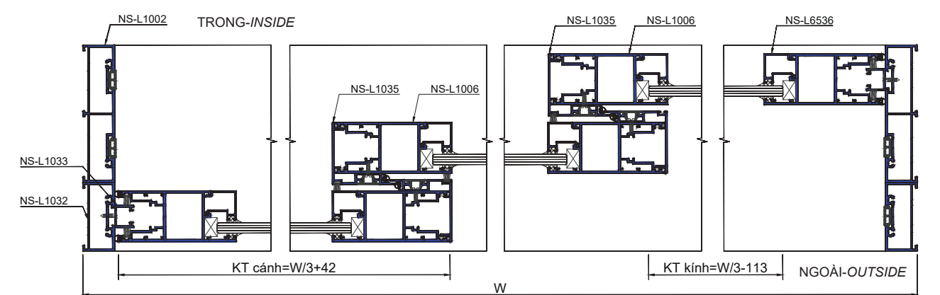
CHI TIẾT 2-2
