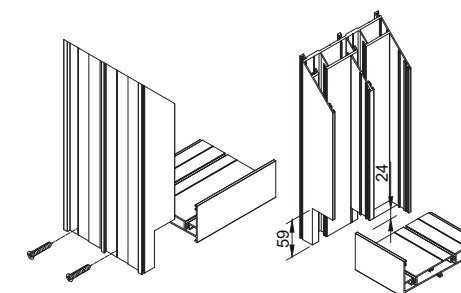
Tham khảo ghép góc ray 90^\circ bằng Vít
