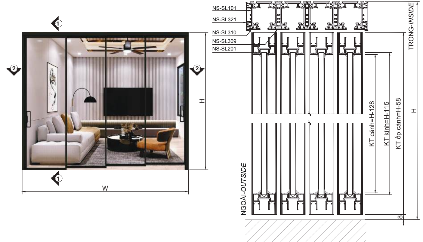
CHI TIẾT 1-1
