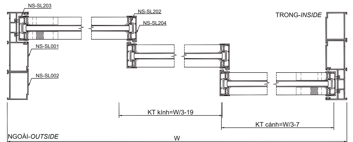
CHI TIẾT 2-2
