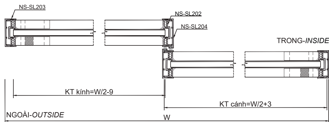
CHI TIẾT 2-2
