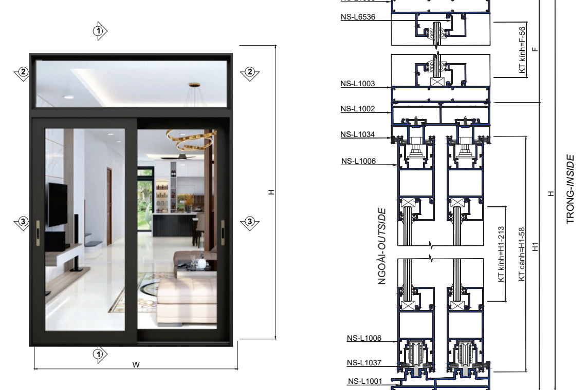
CHI TIẾT 1-1
