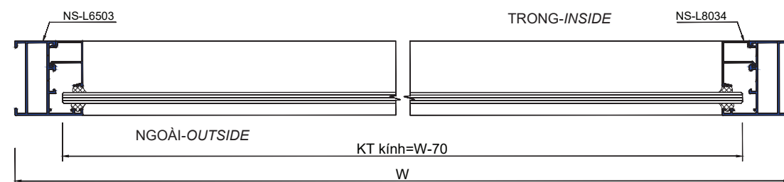
CHI TIẾT 2-2
