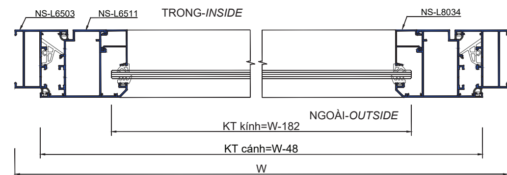
CHI TIẾT 2-2
