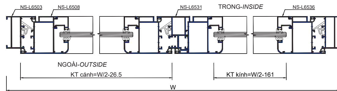
CHI TIẾT 3-3
