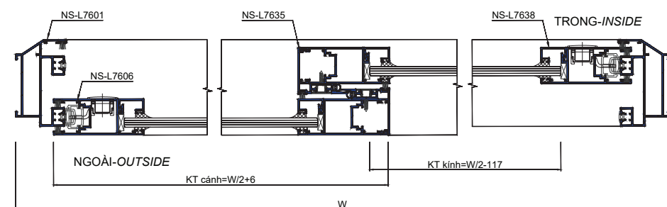
CHI TIẾT 2-2
