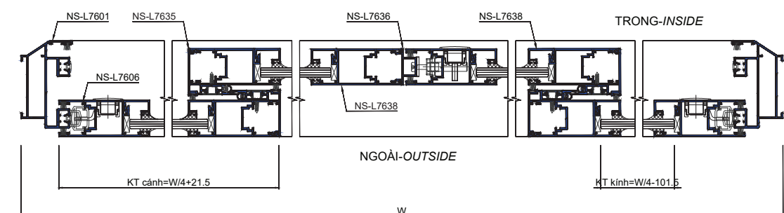
CHI TIẾT 2-2
