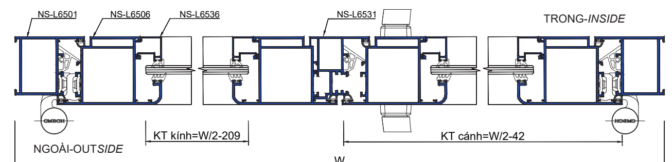
CHI TIẾT 2-2
