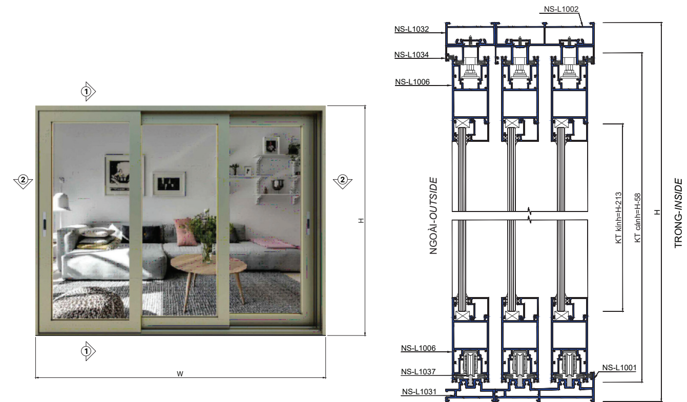
CHI TIẾT 1-1
