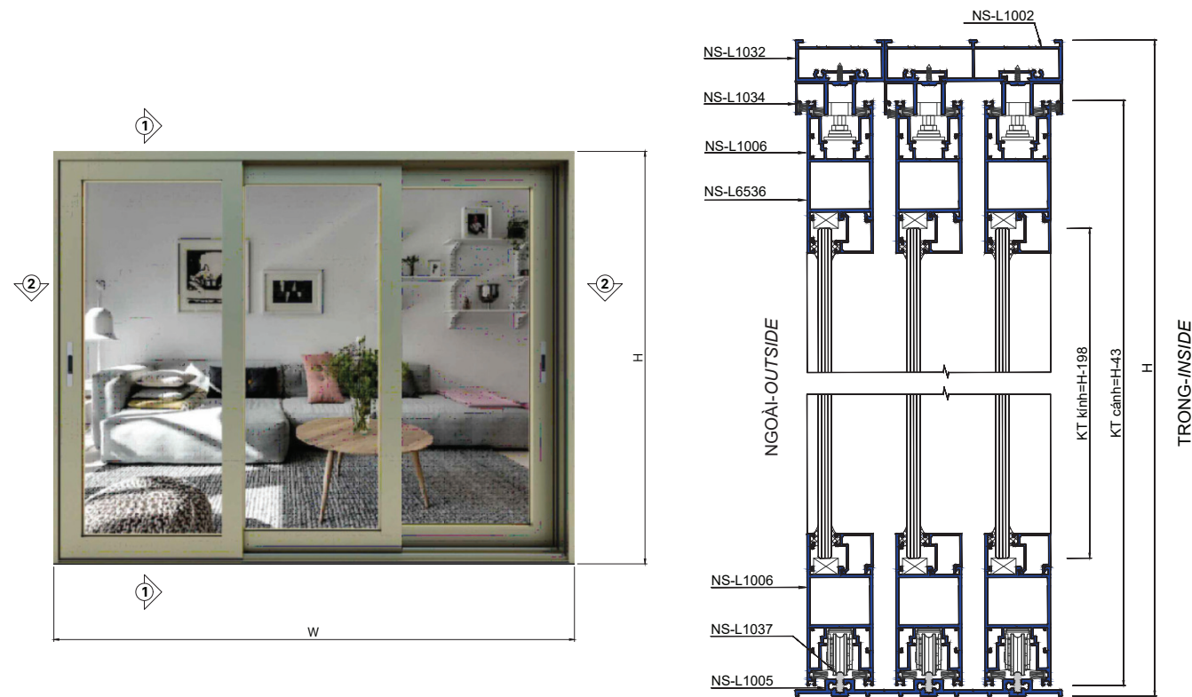
CHI TIẾT 1-1
