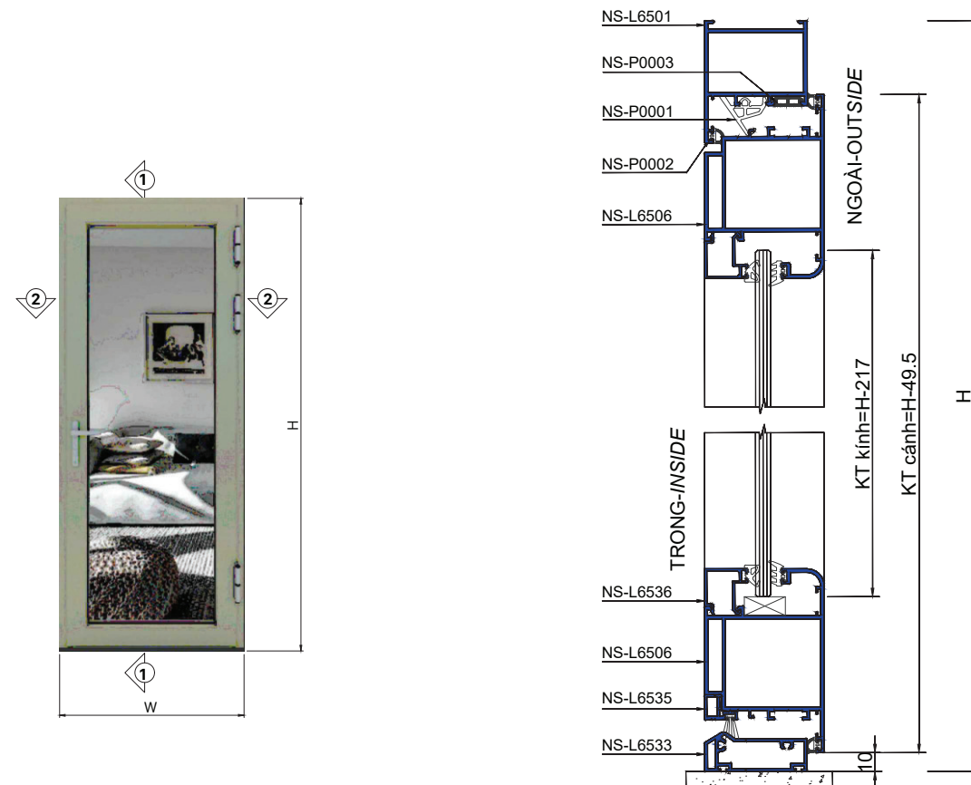
CHI TIẾT 1-1
