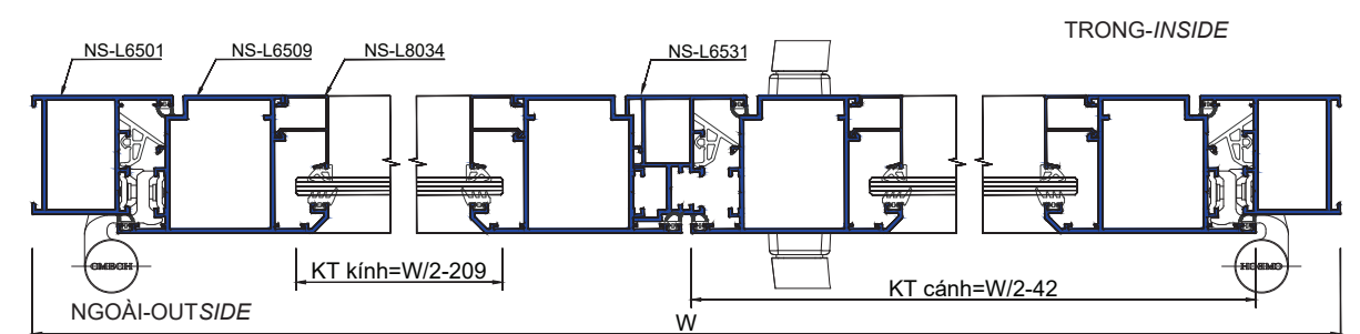
CHI TIẾT 3-3
