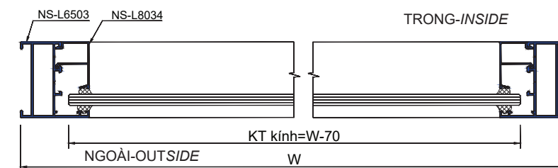
CHI TIẾT 2-2
