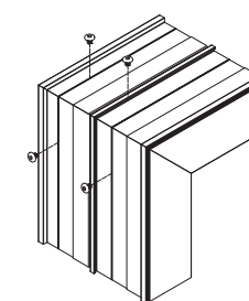
Tham khảo ghép góc cánh 45^\circ ke vĩnh cửu (Vít lục giác)
