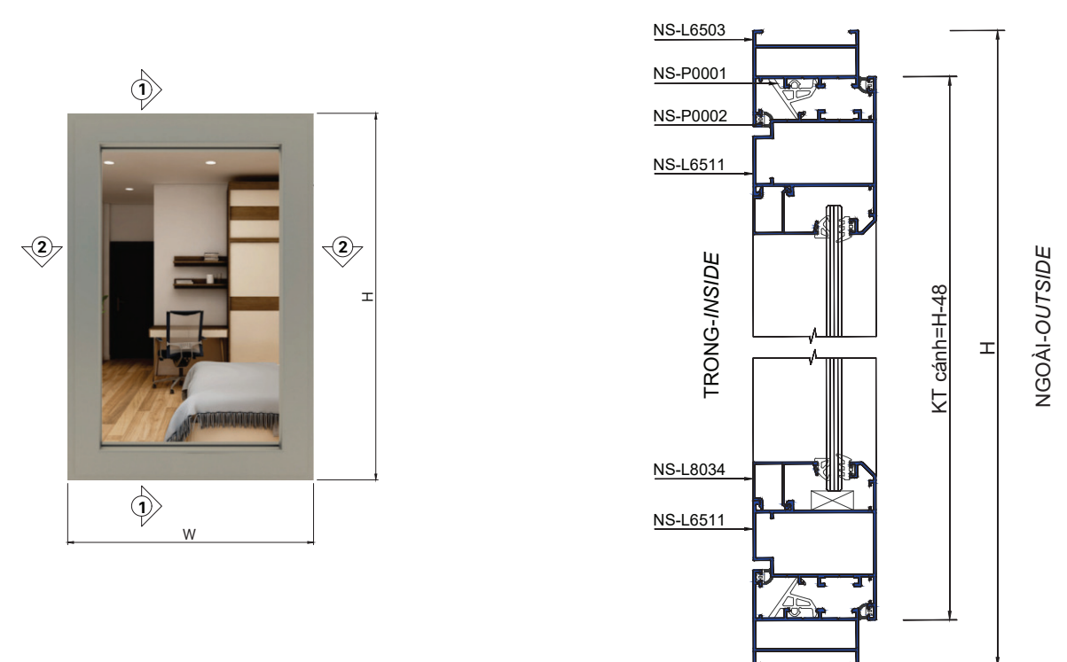
CHI TIẾT 1-1
