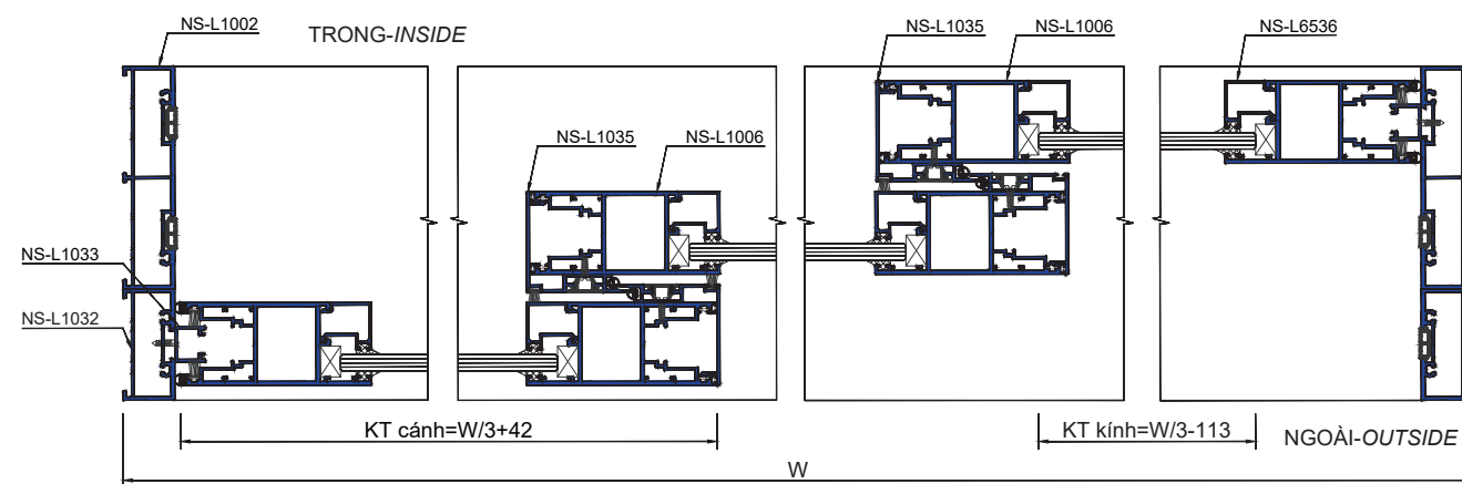
CHI TIẾT 2-2
