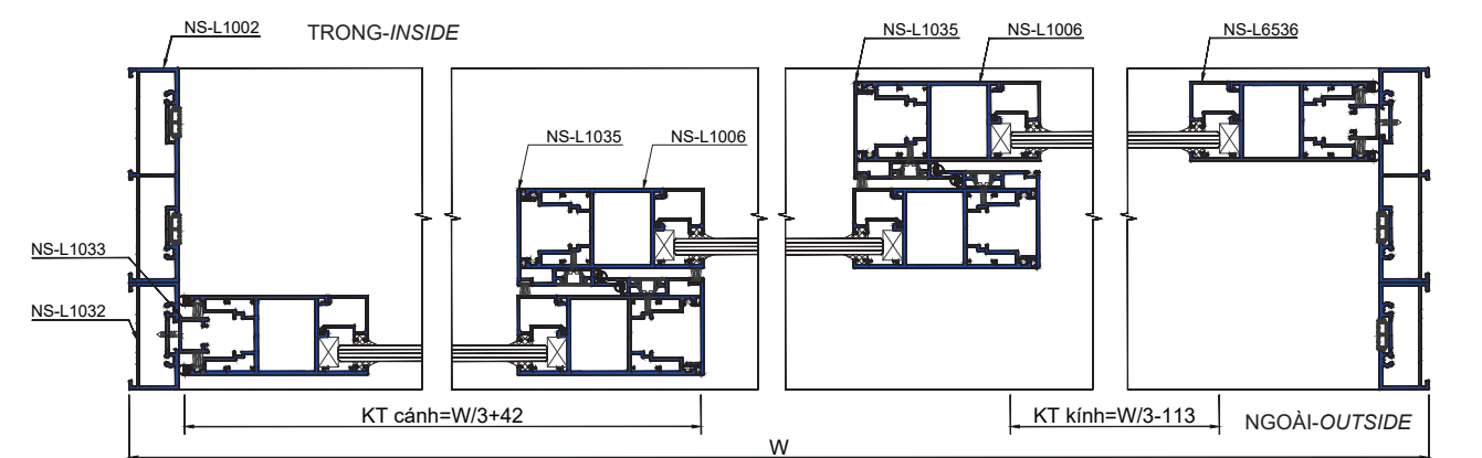
CHI TIẾT 2-2
